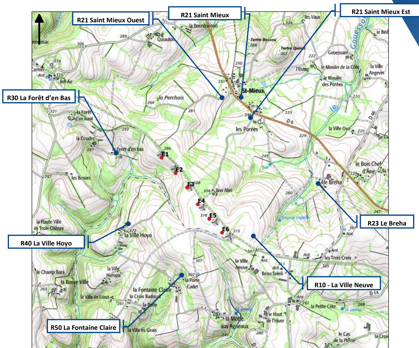
Planche 8 - Localisation des points de contrôle et du projet éolien
