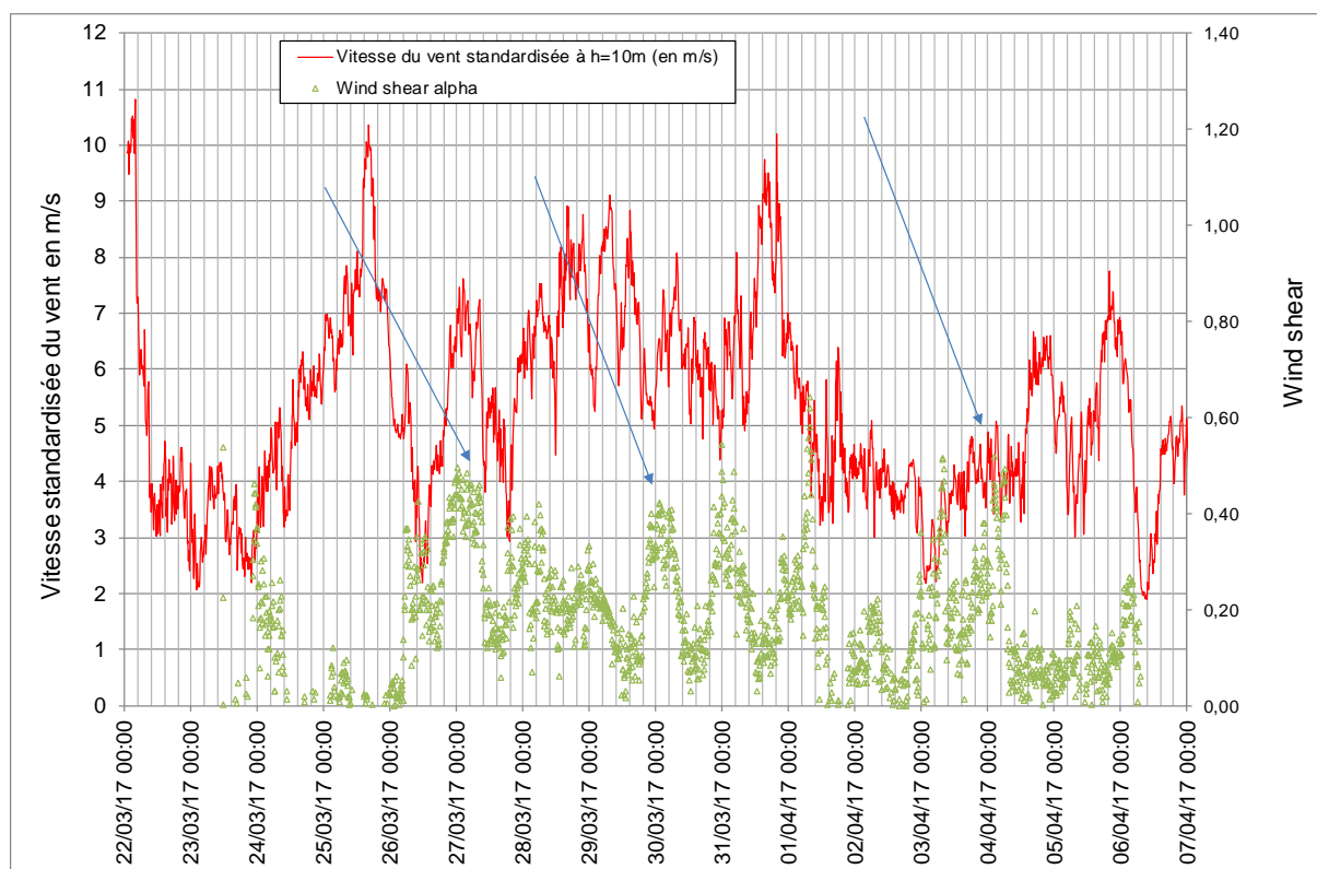
Planche 3 - Vitesses et gradients de vent
