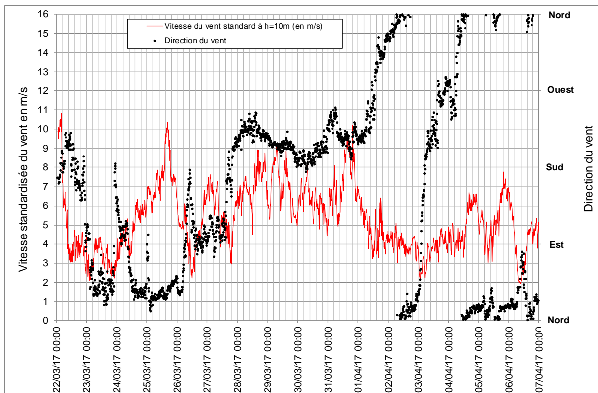
Planche 2 - Relevés météorologiques du 22 mars au 6 avril 2017
