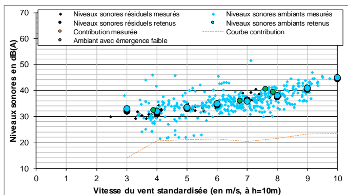
Vent de Sud-Ouest [135° - 315°]
